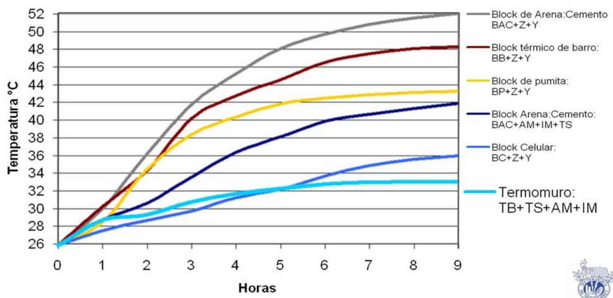
Exposición a Temperatura Constante de 70°C (Día de verano a 40 °C)
